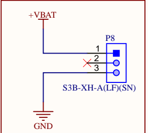
Connector JST
