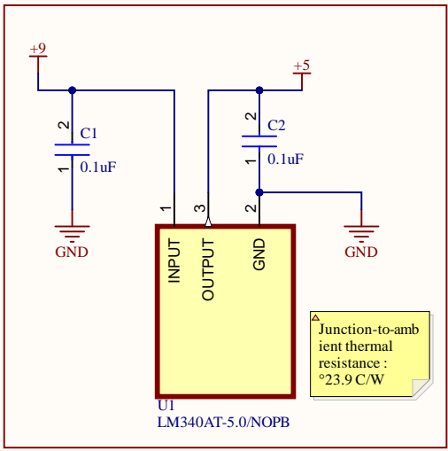
Régulateur 5V
